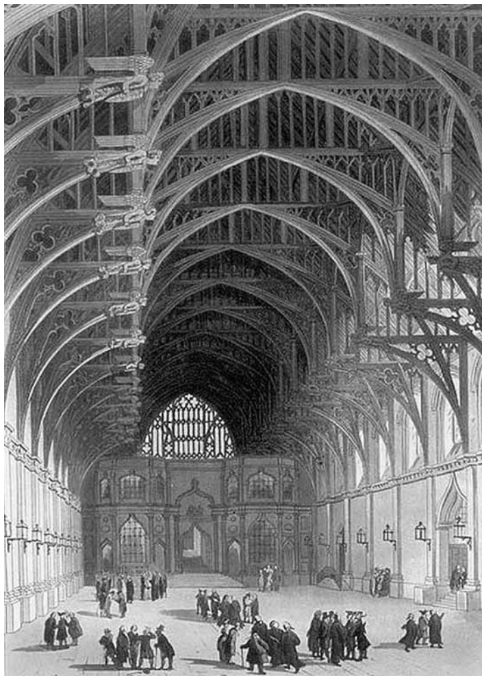
Na obraze Westminster Hall z roku 1808 je dobře vidět nezvyklá vazba, kterou na konci 14. století vytvořil královský tesař Hugh Herland. Využil principu vzpěry a všadla se mu vyloučit vazné trámy. Na počátku 19. století tento typ konstrukce technicky popsal a zdokonalil francouzský inženýr Paul Ardant, po němž se této soustavě říká „Ardantova“. Dříve se používala k zastřešení velkých prostor o šířce 20 a více metrů. Foto: archiv autora.
