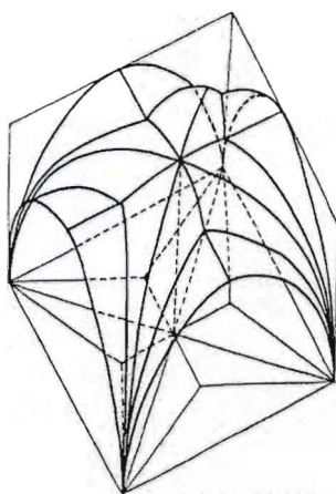
klenba, (hvězdová)
